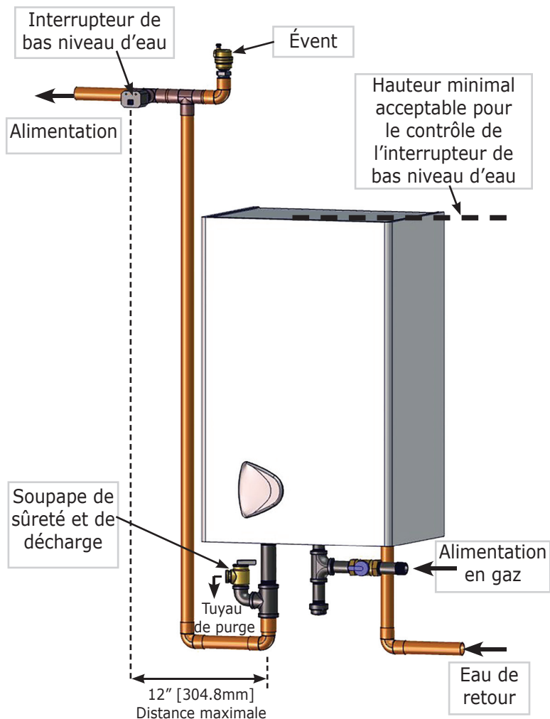
Figure 10 - Localisation possible de la sonde de l'interrupteur de bas niveau d'eau
