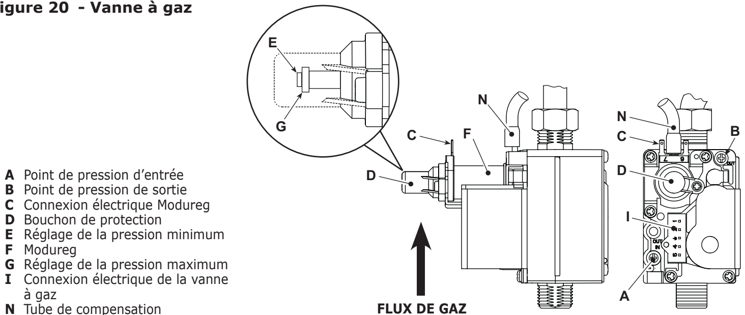
Figure 20 - Vanne à gaz
