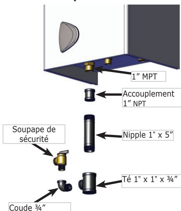
Figure 8 - Soupape de sécurité et évent d'air (vue de face à la chaudière)
