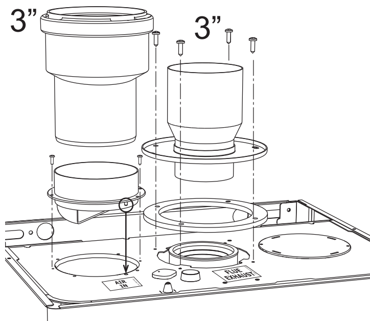
Figure 12 - Raccord d'air de combustion
