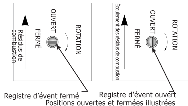
Figure 3 – Indicateur de position du registre d'évent
