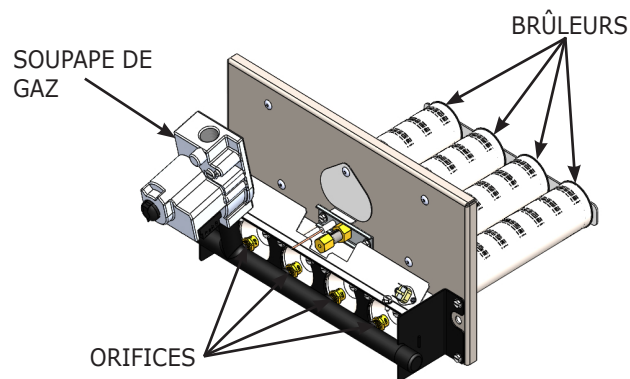
Figure 14-1 – Plateau du brûleur
