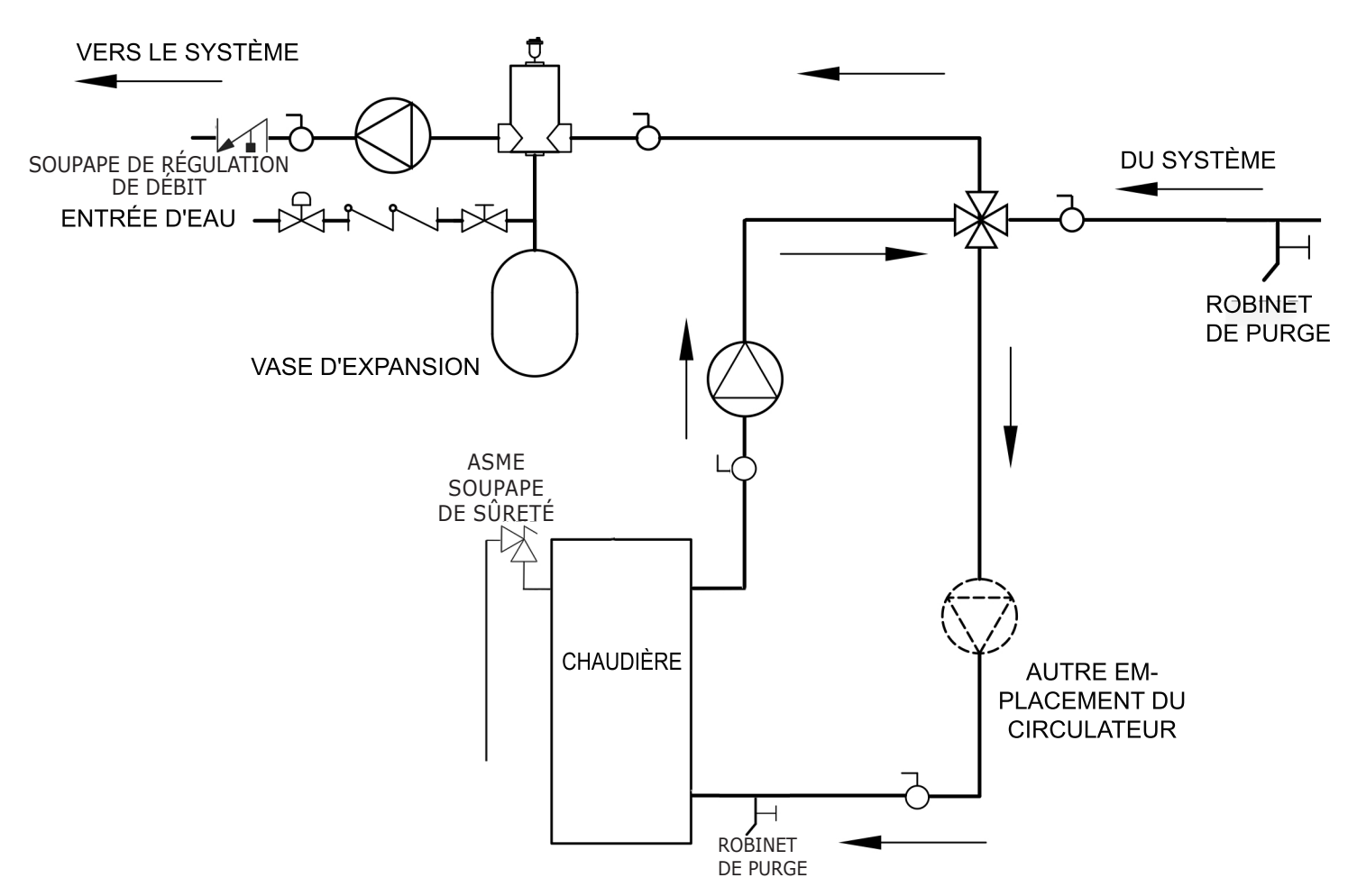
Figure 4-7 – Canalisation de dérivation (option de soupape à 4 voies avec circulateur du côté de l'alimentation)
