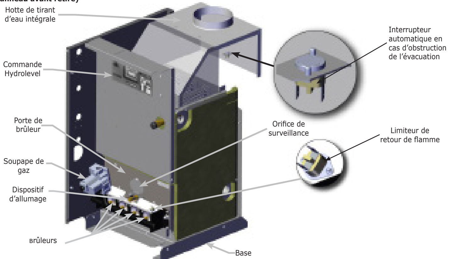
Figure 13-1 Interrupteur manométrique en cas d'obstruction de l'évacuation, limiteur de retour de flamme (panneau avant retiré)
