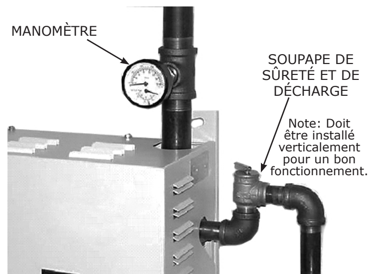
Figure 1A - Soupape de sûreté et de décharge
