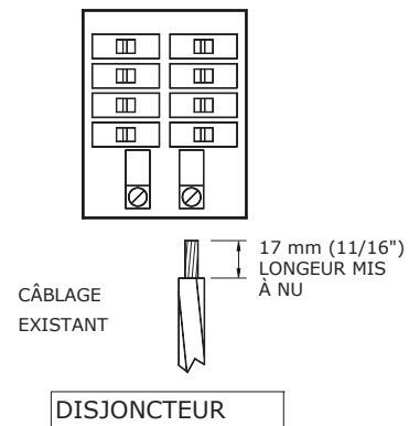
Figure 5 - Schéma de câblage
