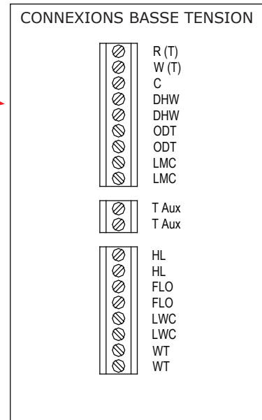
Figure 8 - Câblage basse tension du panneau de contrôle Board
