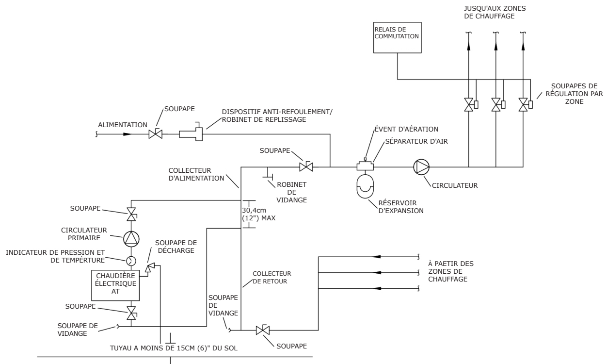
Figure 3 - Conduits primaires/secondaires pour zones multiples et soupapes de régulation par zone
