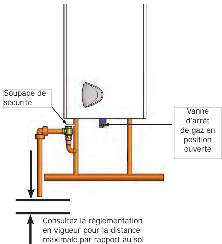
Figure 8 - Tuyauterie d'évacuation de la soupape de sécurité
