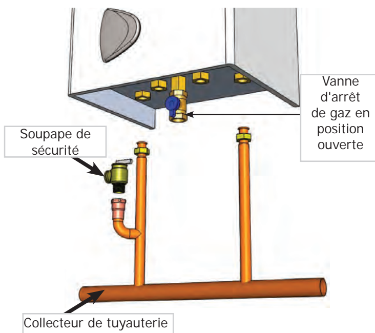
Figure 7 - Soupape de sécurité et évent d'air (vue de face à la chaudière)
